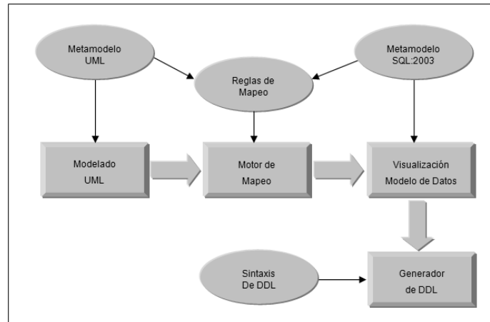
Fig. 8. Esquema general de la herramienta OR-Transformer
