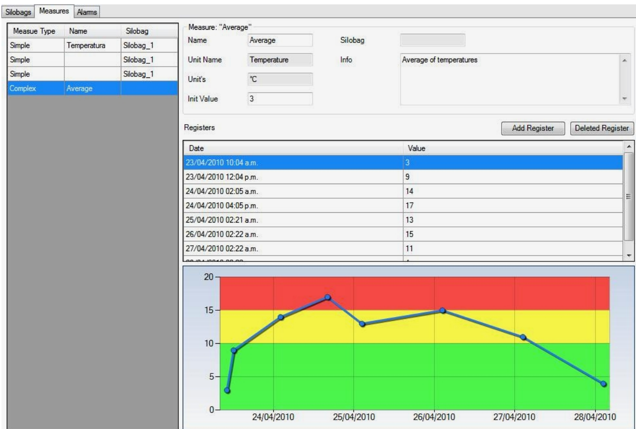
Figura 7: Interfaz con medidas y resultado de registros
