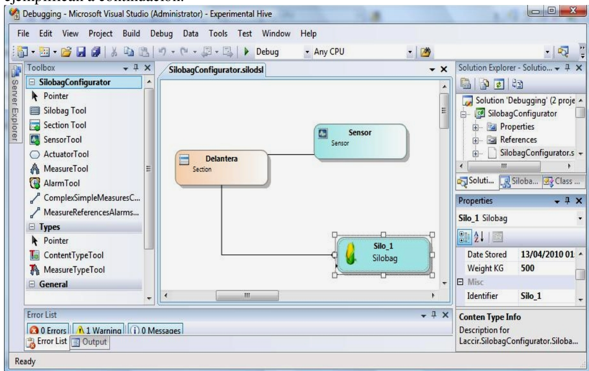
Figura 3: Editor del DSL
