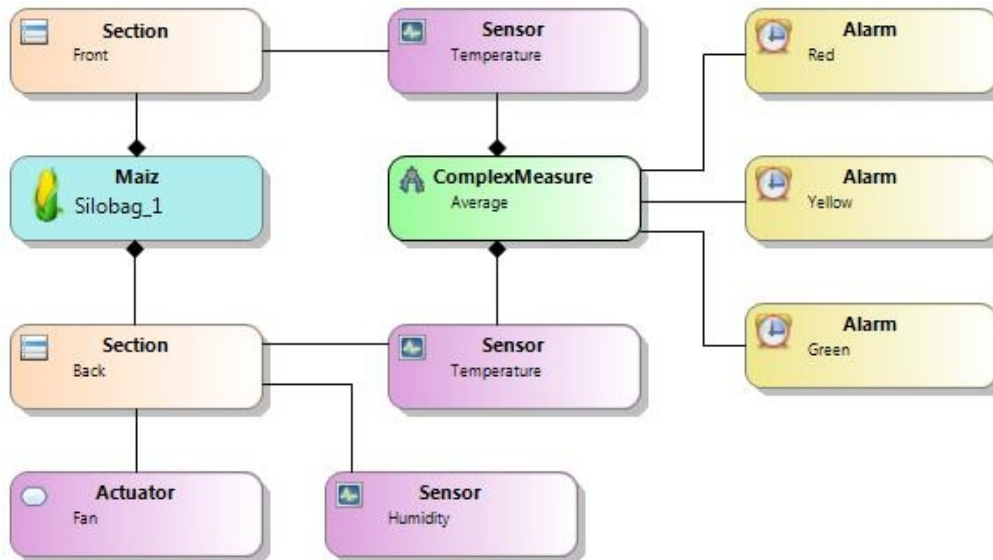
Figura 4: Configuración utilizando el DSL
