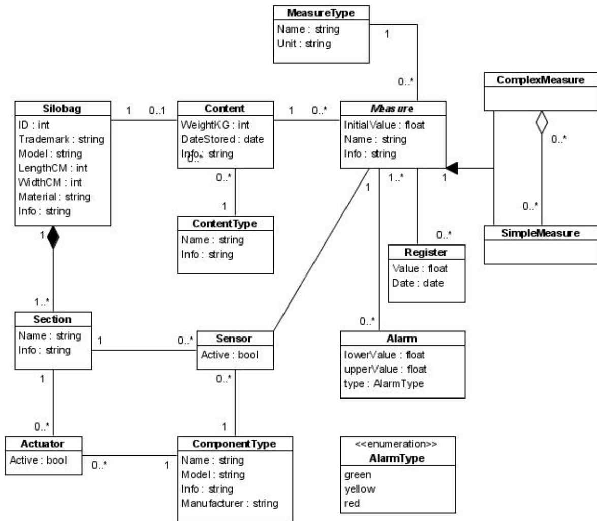
Figura 2: Meta-Modelo del DSL
