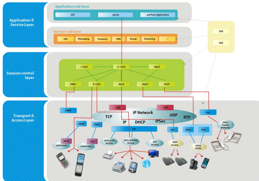
Figura 1: Arquitectura IMS
