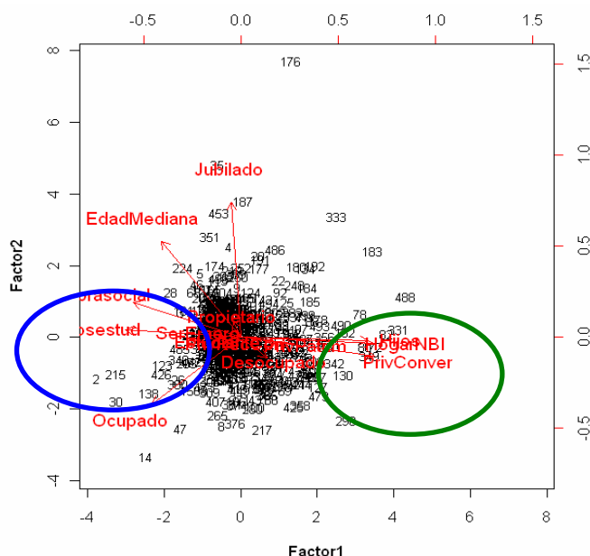
Figura 1: Biplot de los dos primeros factores
